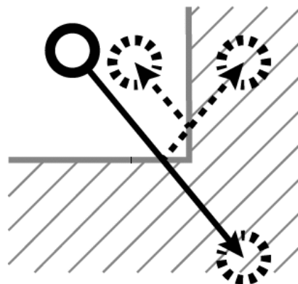
Slika 2. Moguća komplikacija prilikom sudara čestice sa preprekom
