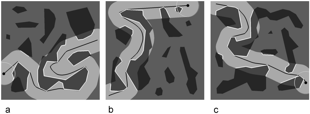
Slika 17. Rezultati implementacije
