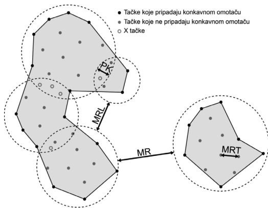
Slika 1. Proces generisanja terana
