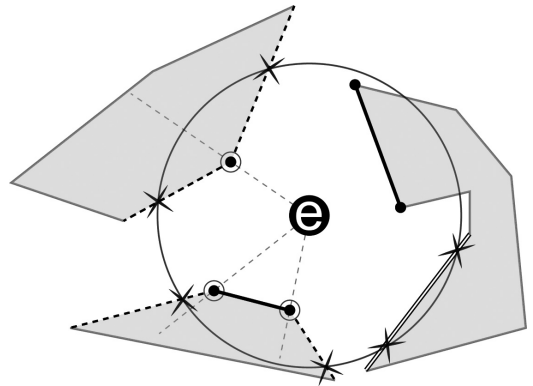
Slika 7. Ažuriranje PNOD-ova
