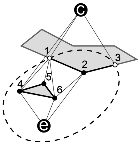
Slika 14. Primer grafa povezanosti nodova u okviru istražene površine
