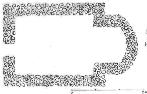
Slika 1. Tlocrt crkve na groblju u selu Mazgoš (crtež: K. Celner)
